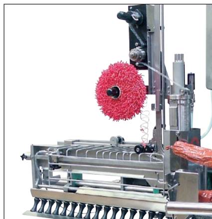
Dispositivo de alimentación para lazos de embutido
