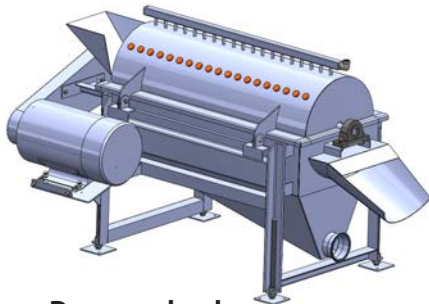
Desgrasador de mollejas GD-T
