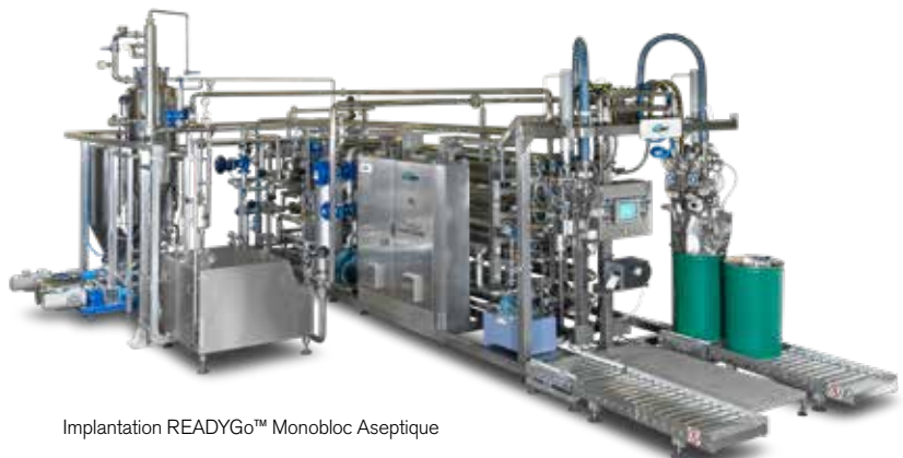
Remplisseuses aseptiques
